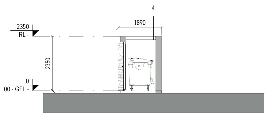
8 Section A-A 1:100
